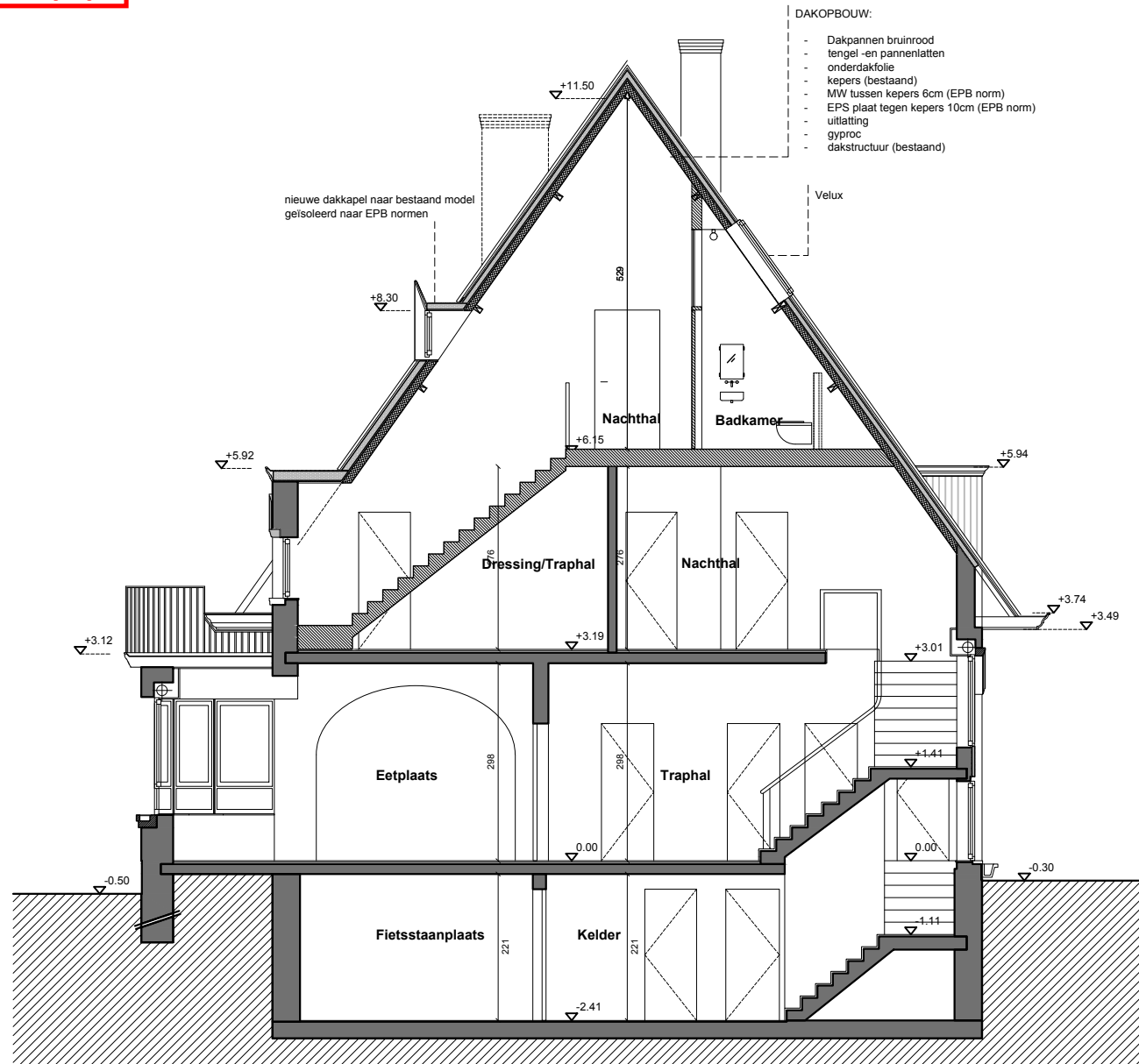
SNEDE AA'
