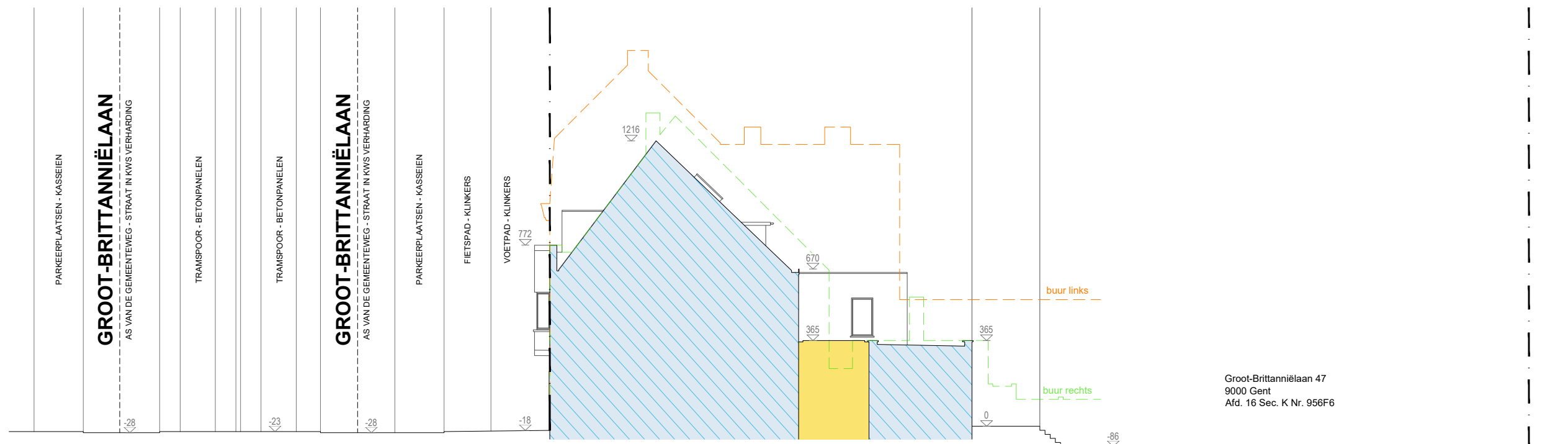
Terreinprofiel Nieuwe toestand Schaal 1/200
