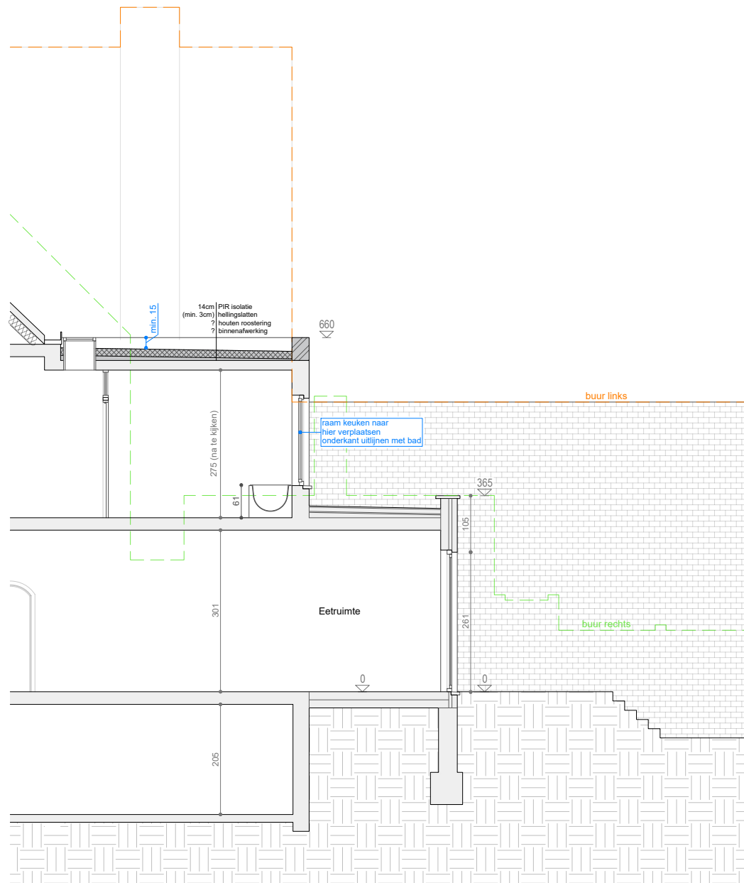
Snede BB Nieuwe toestand Schaal 1/100
