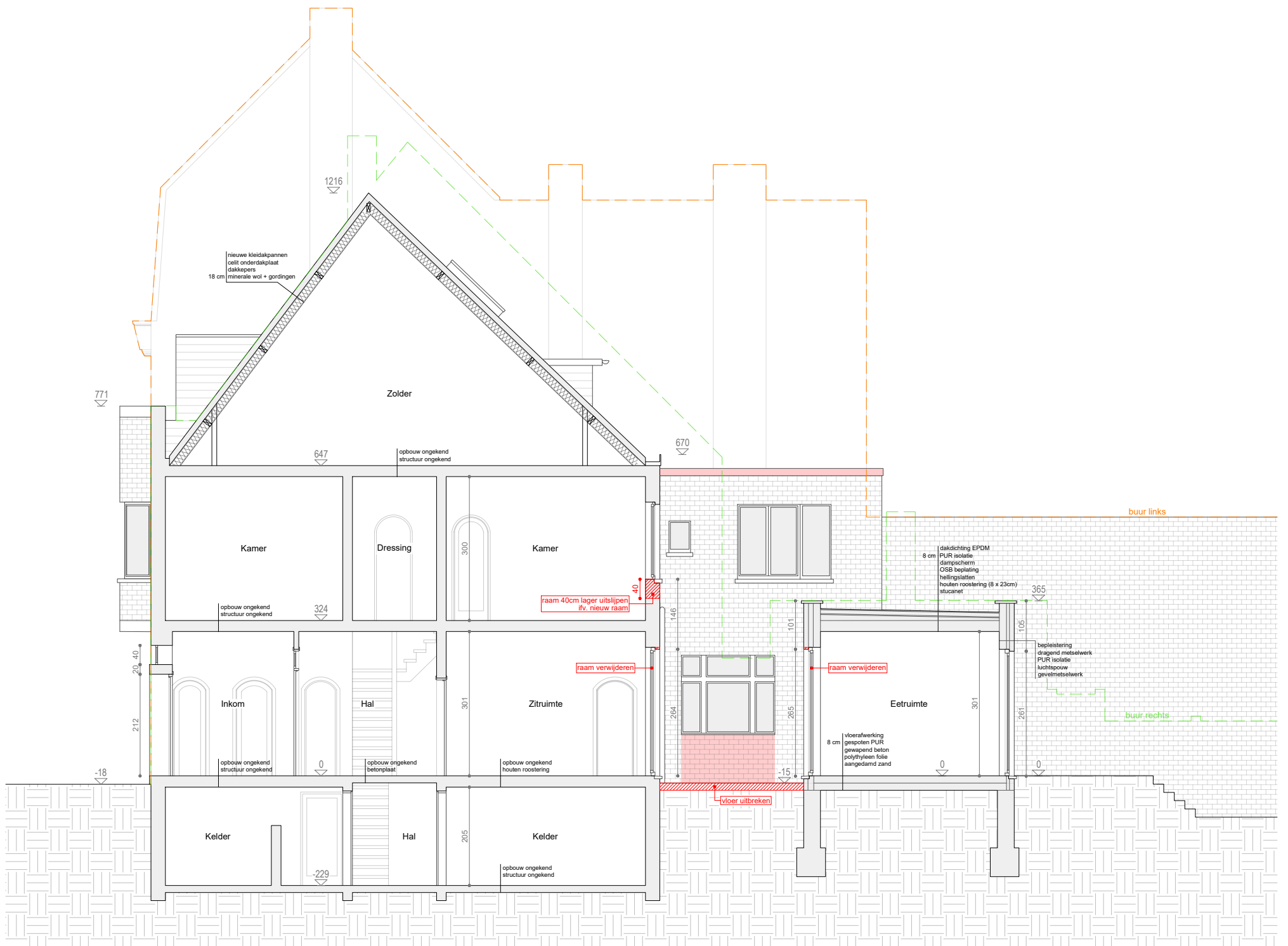
Snede AA Bestaande toestand Schaal 1/100
