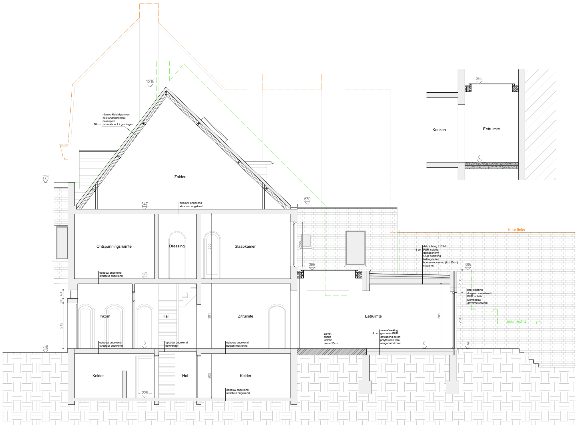
Snede AA Nieuwe toestand Schaal 1/100
