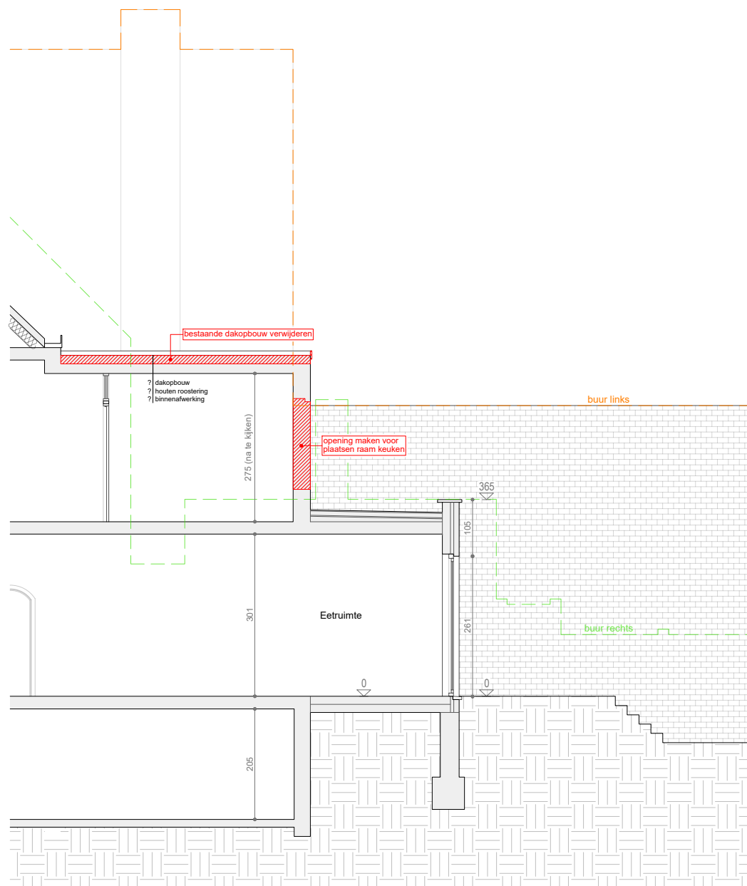
Snede BB Bestaande toestand Schaal 1/100
