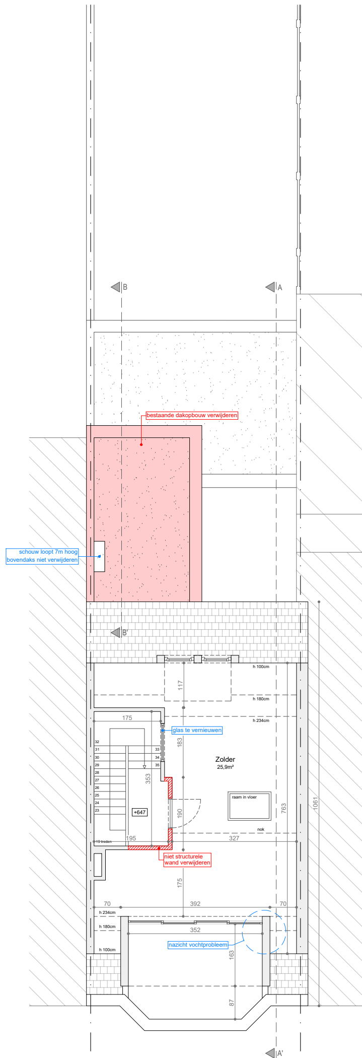
Verdieping +2 Bestaande toestand Schaal 1/100
