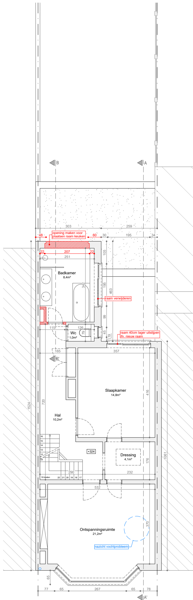
Verdieping +1 Bestaande toestand Schaal 1/100
