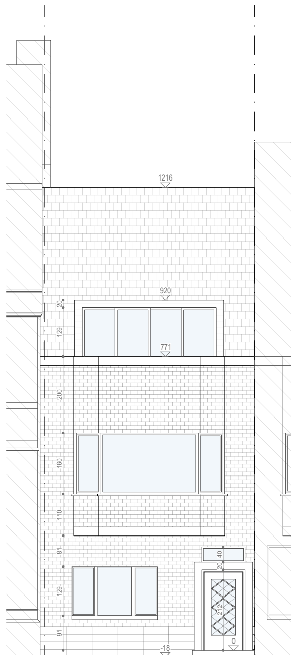
Voorgevel Nieuwe toestand Schaal 1/100
