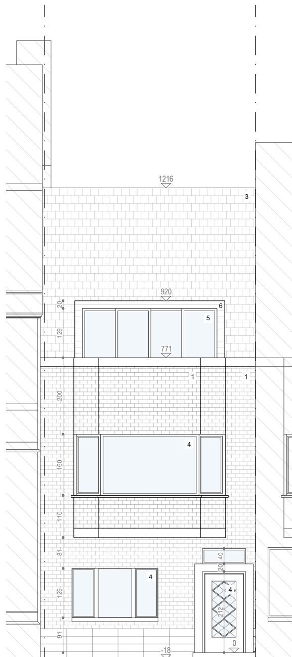
Voorgevel Bestaande toestand Schaal 1/100
