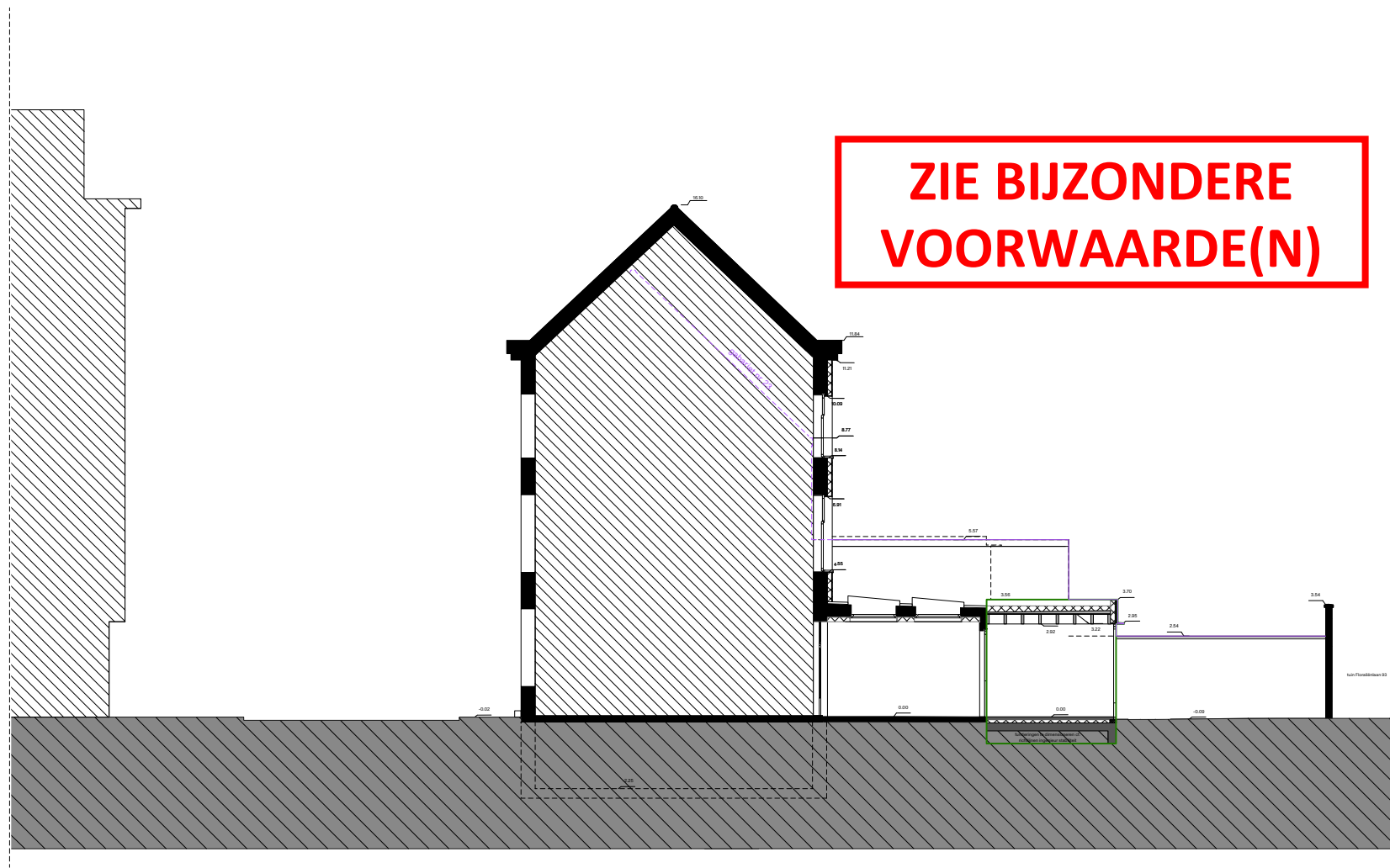
NIEUWE TOESTAND terreinprofiel B schaal 1:200
