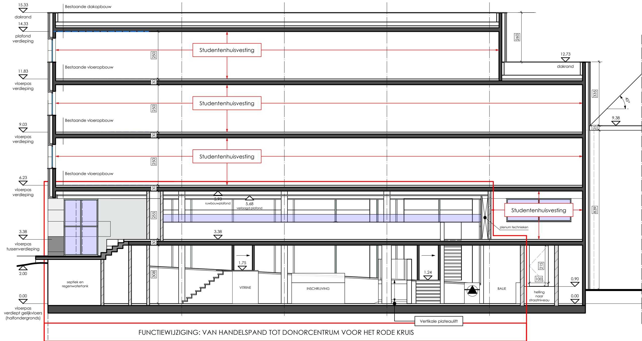
Doorsnede BB S_N_2 Schaal: 1:100
