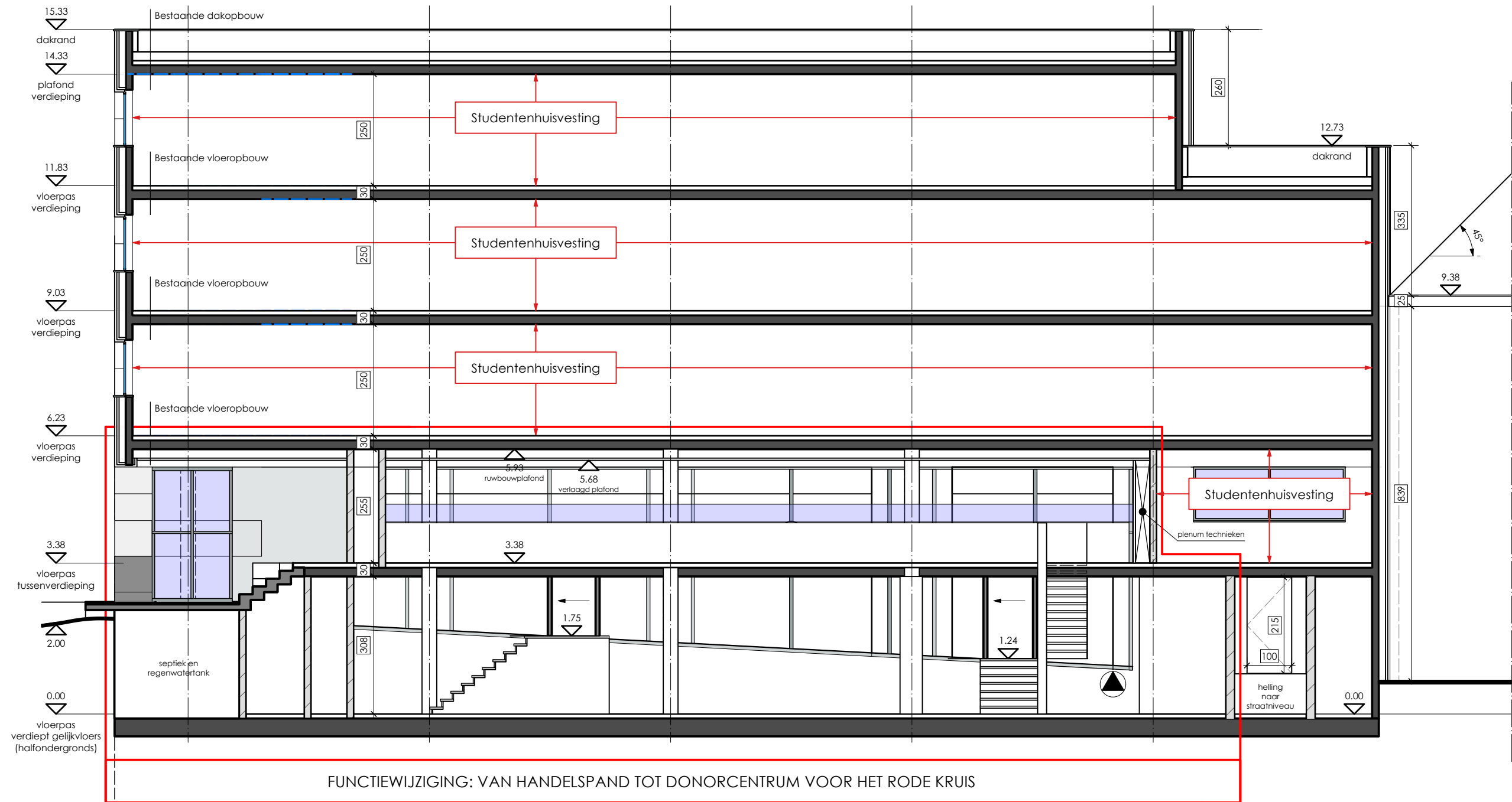
Doorsnede BB S_B_2 Schaal: 1:100
