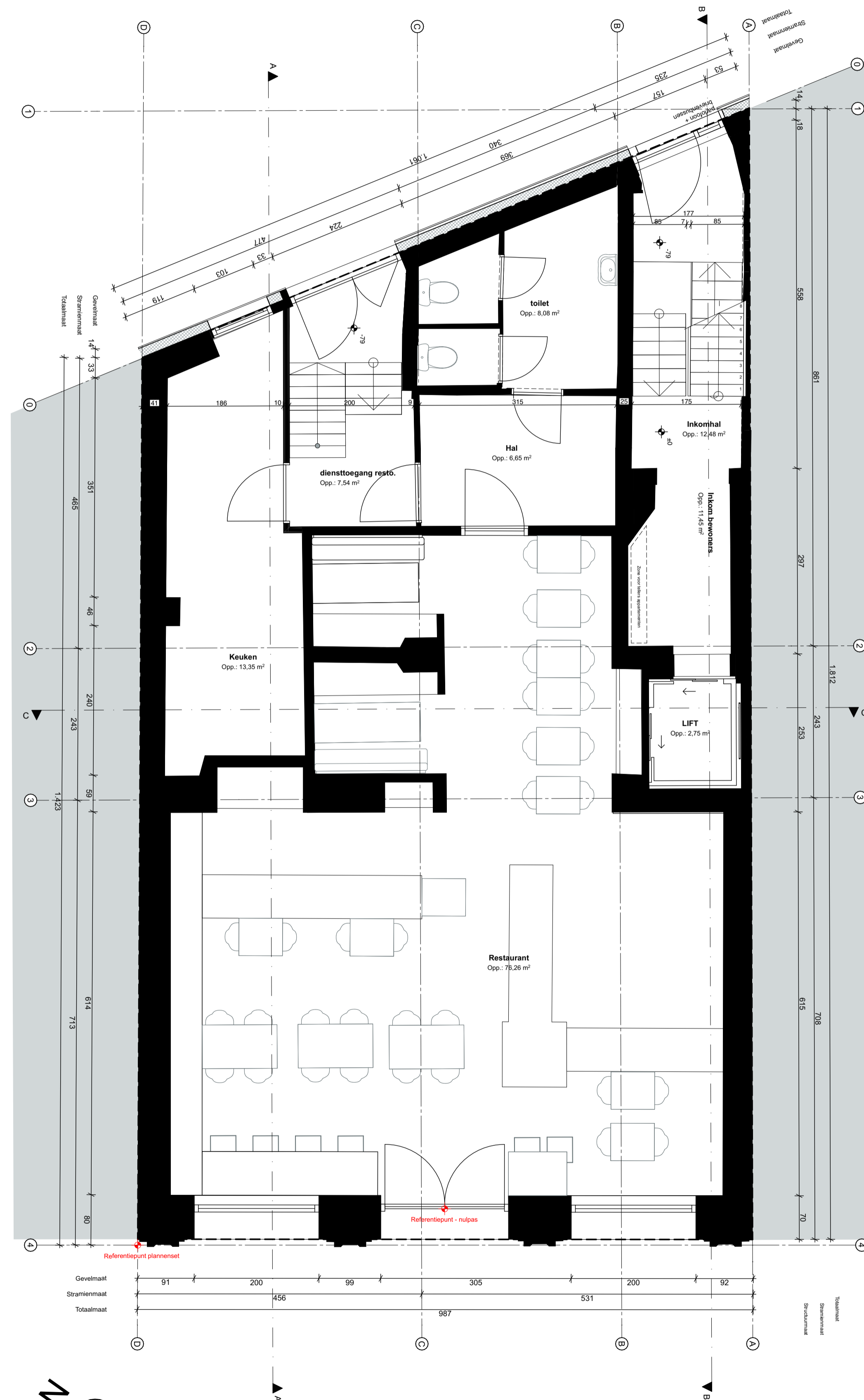
NT - GRONDPLAN GELIJKVLOERS
