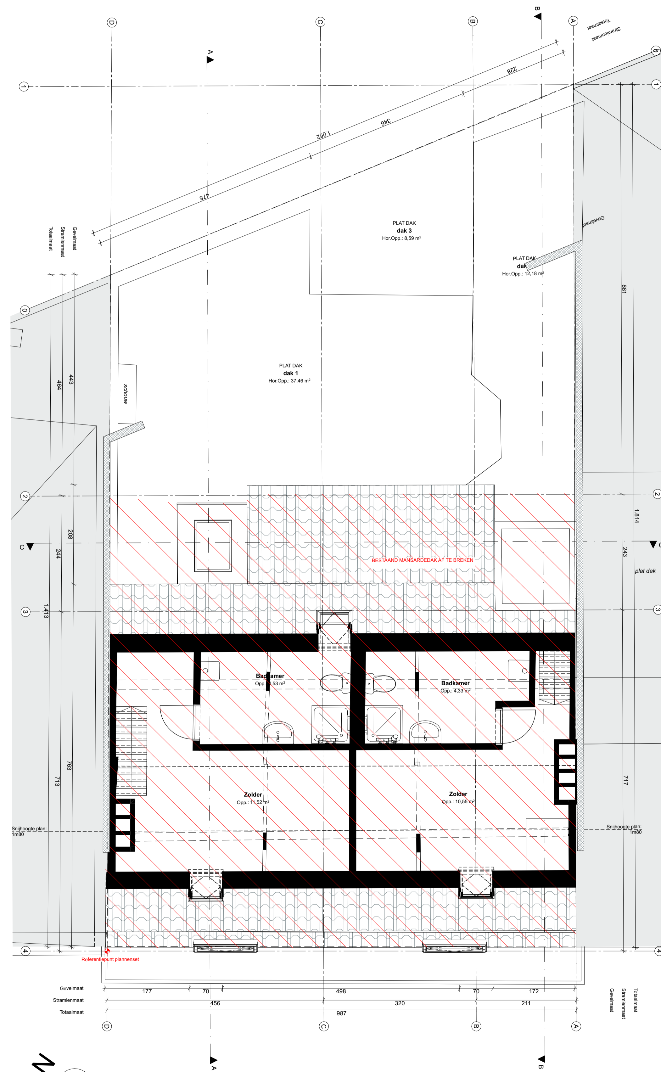
BT - GRONDPLAN +4
