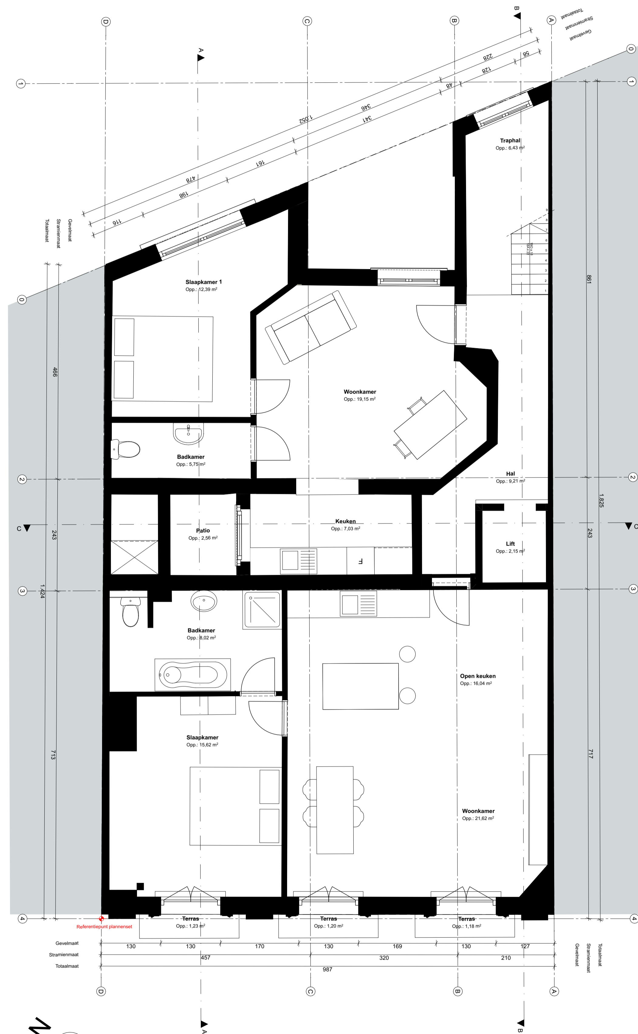
BT - GRONDPLAN +2
