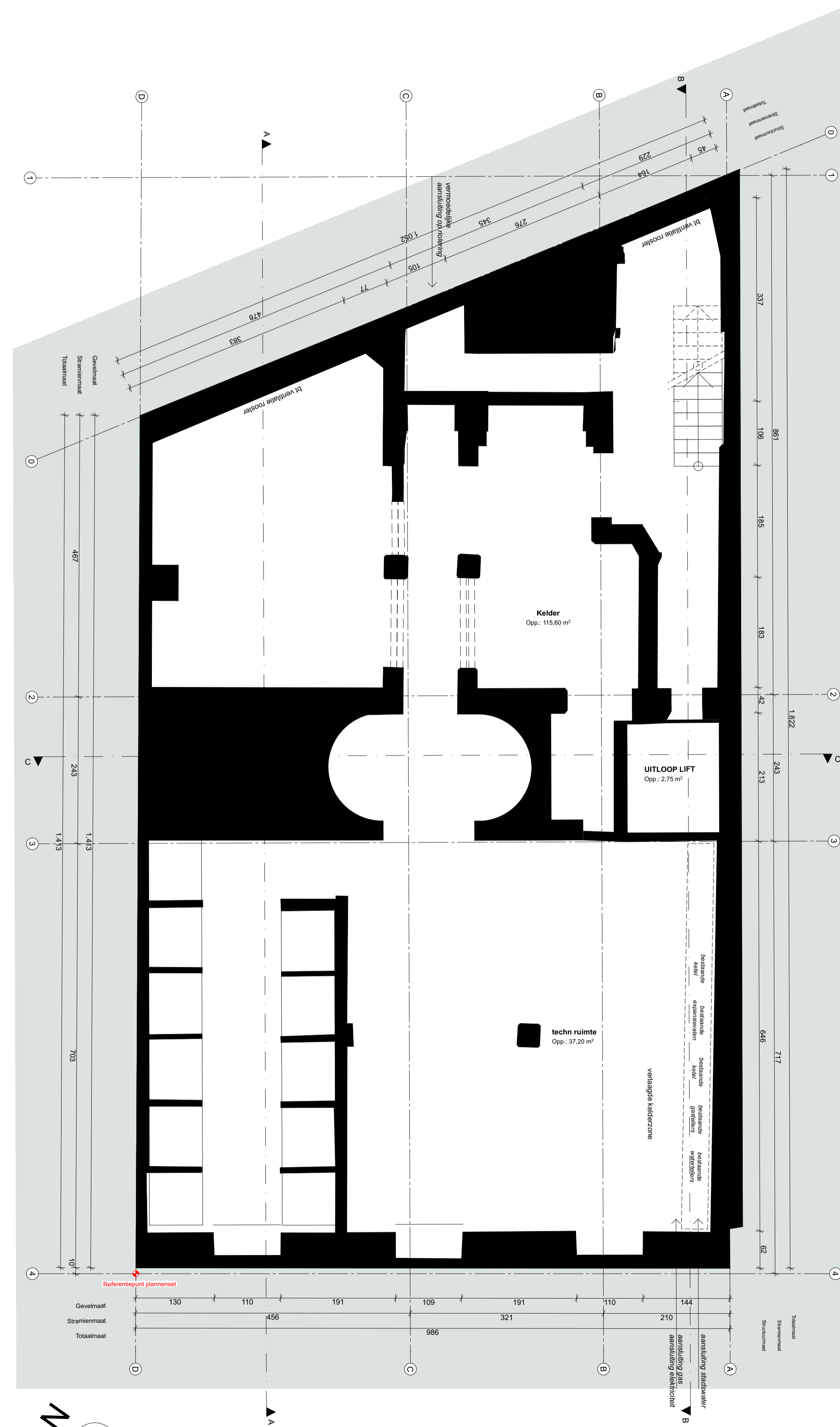
BT - GRONDPLAN KELDER
