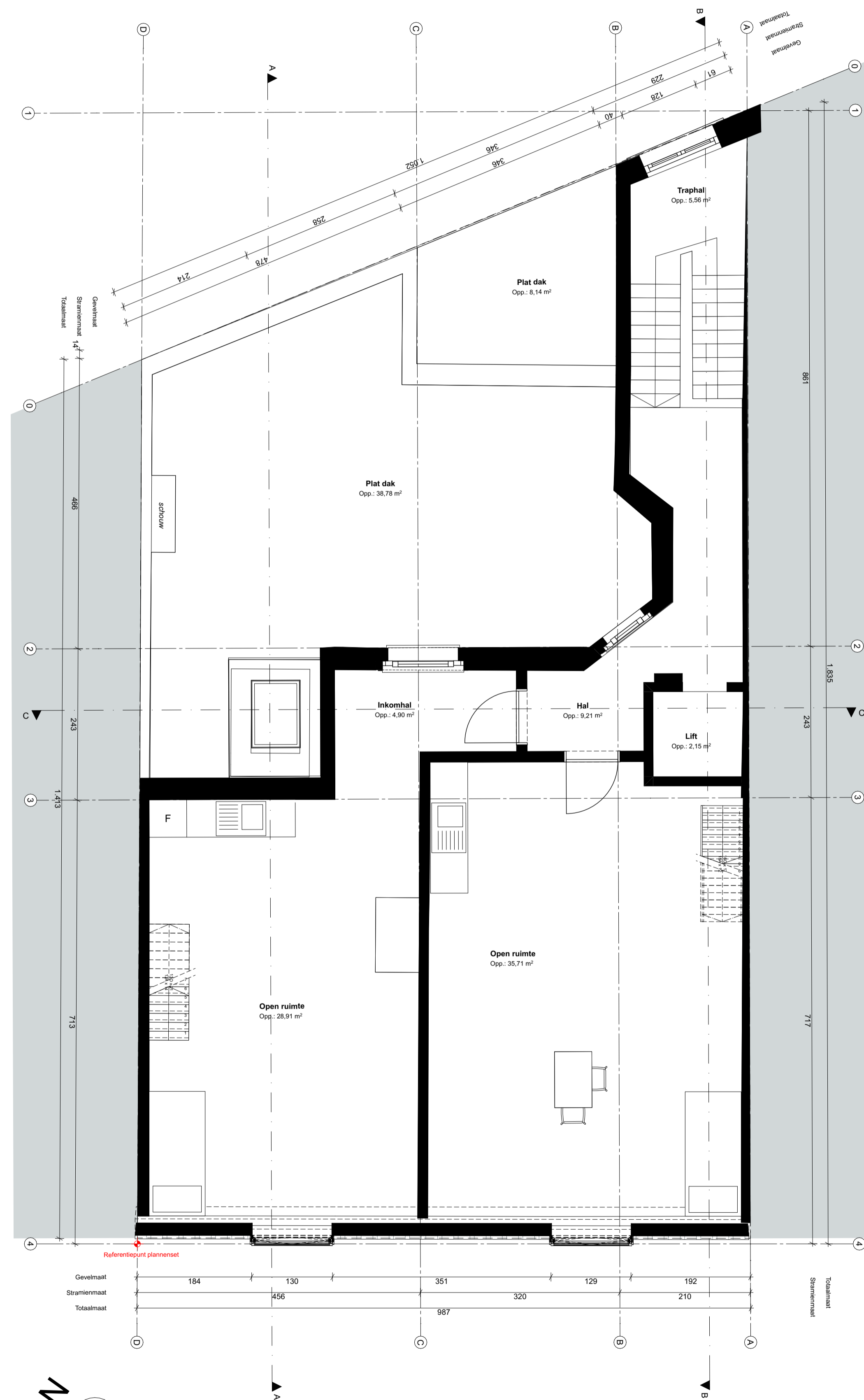
BT - GRONDPLAN +3
