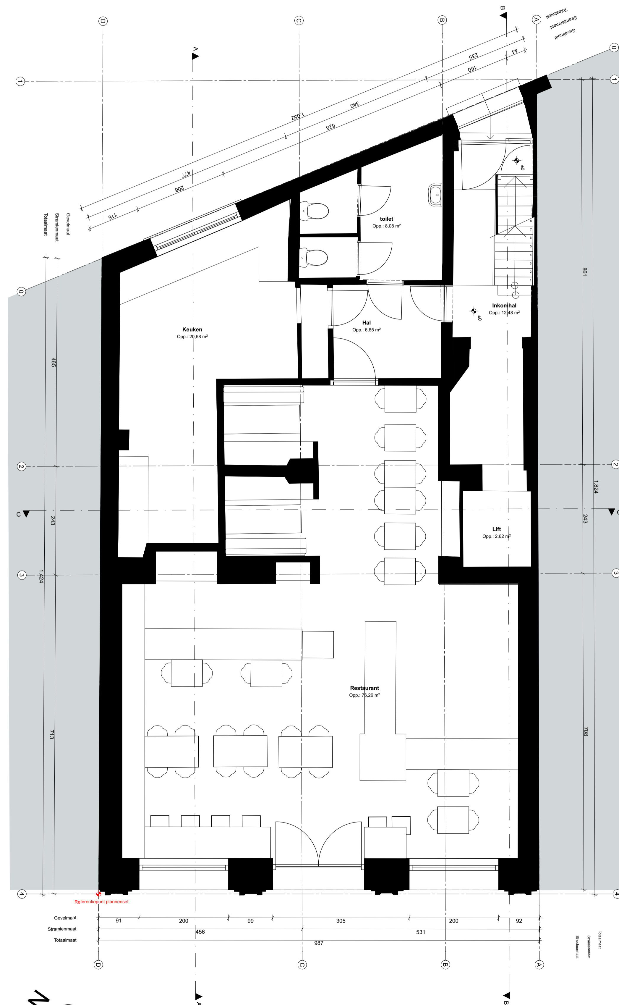
BT - GRONDPLAN GELIJKVLOERS
