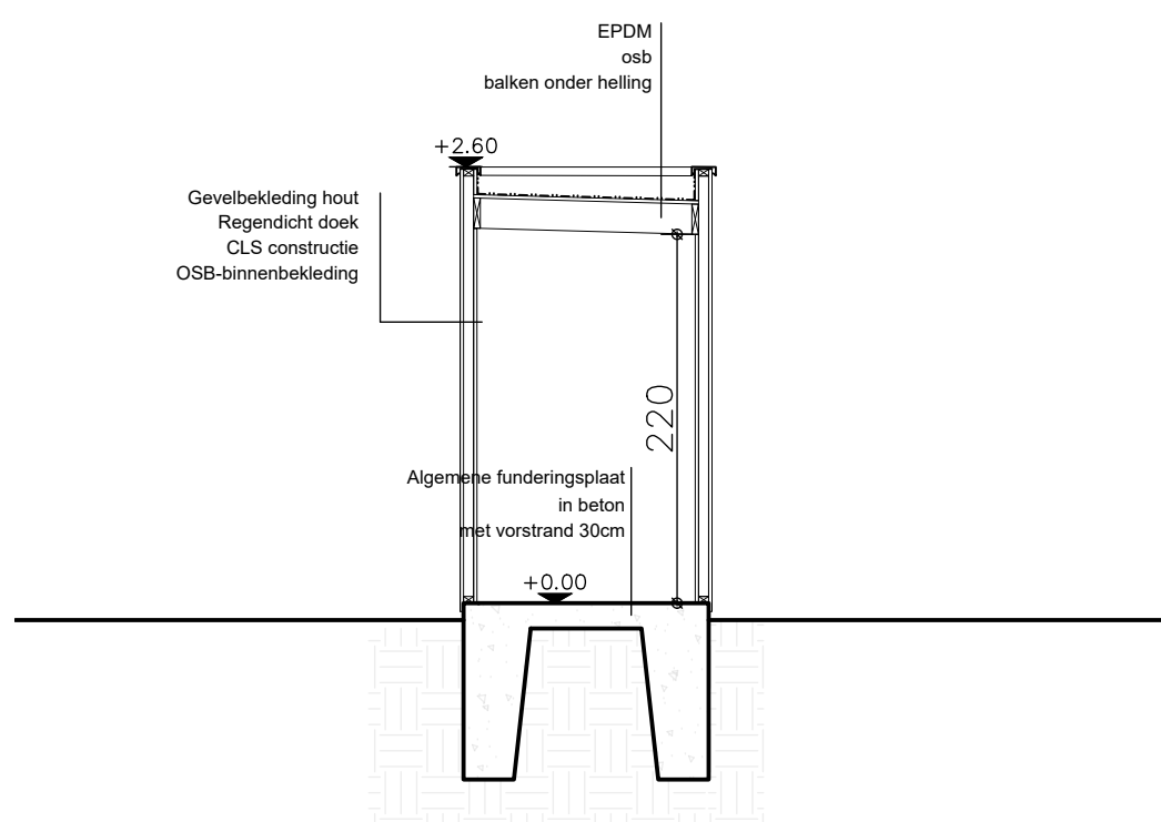
DOORSNEDE AA TUINBERGING NIEUWE TOESTAND
