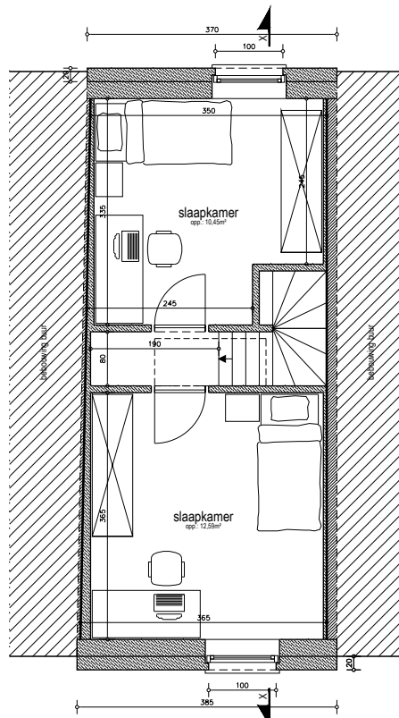
dakverdieping nieuwe toestand
