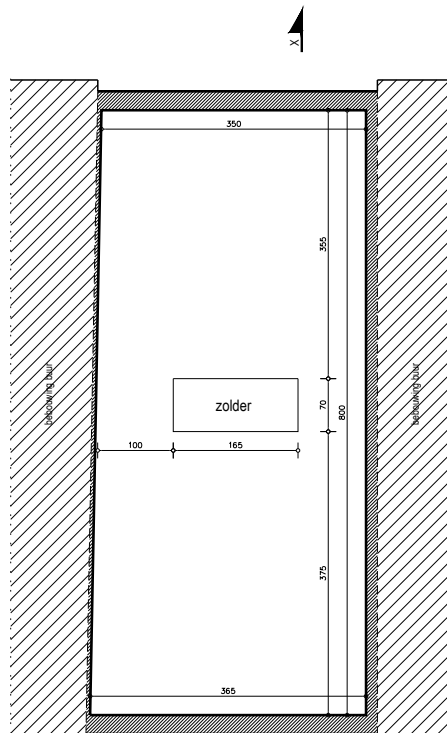
dakverdieping bestaande toestand
