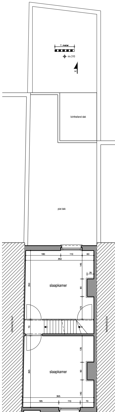
verdieping bestaande toestand
