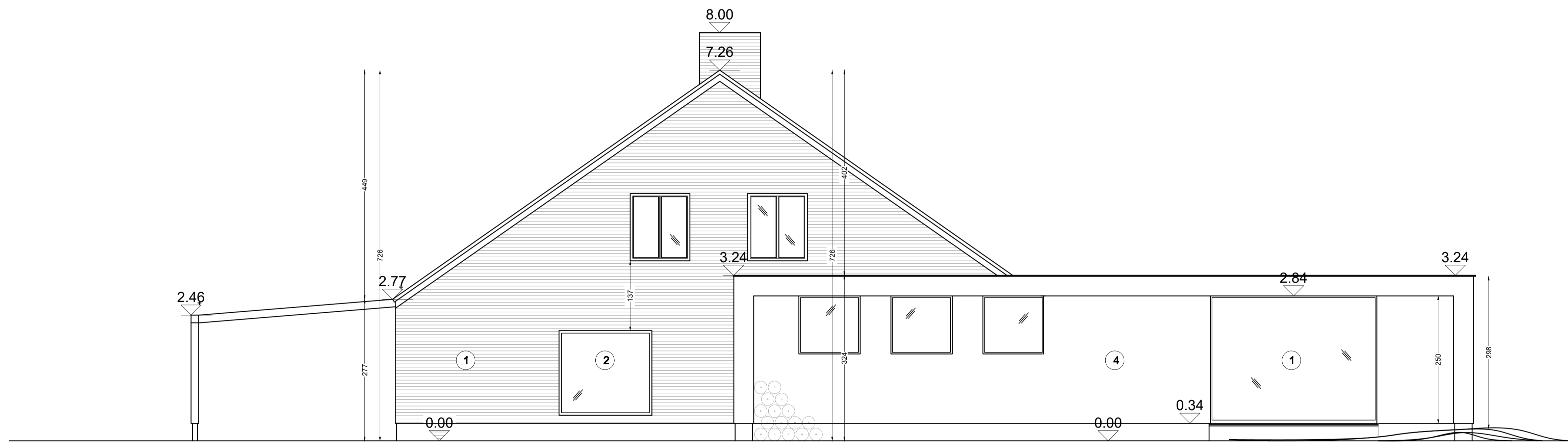
Gevel links Vergunde toestand
