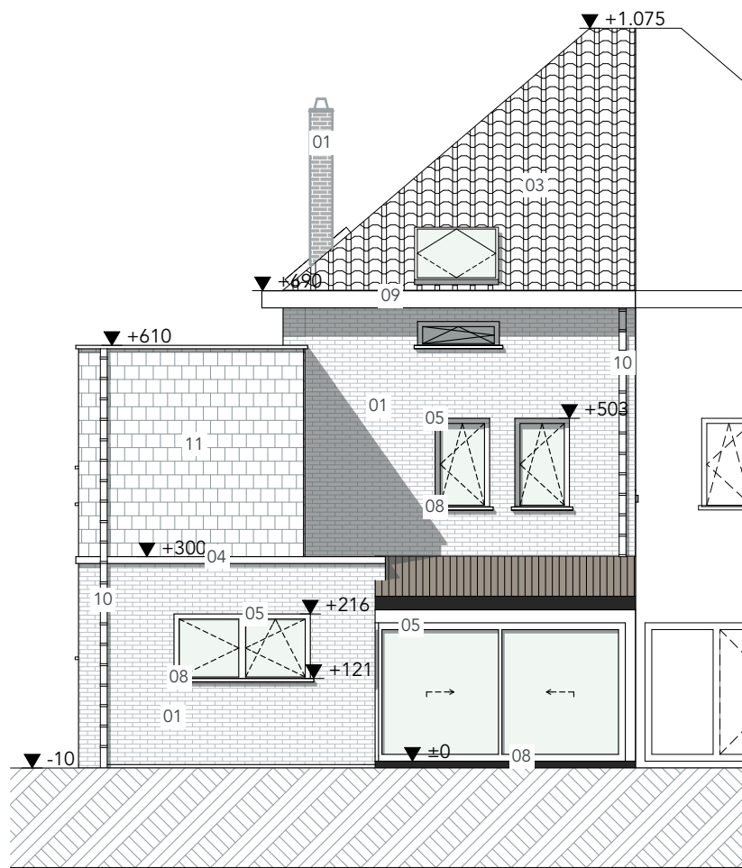
0 1 2 3 4 NT Achtergevel
