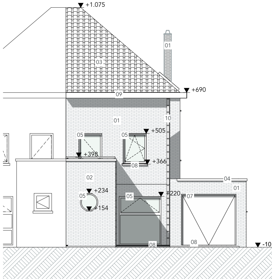
BT Voorgevel
