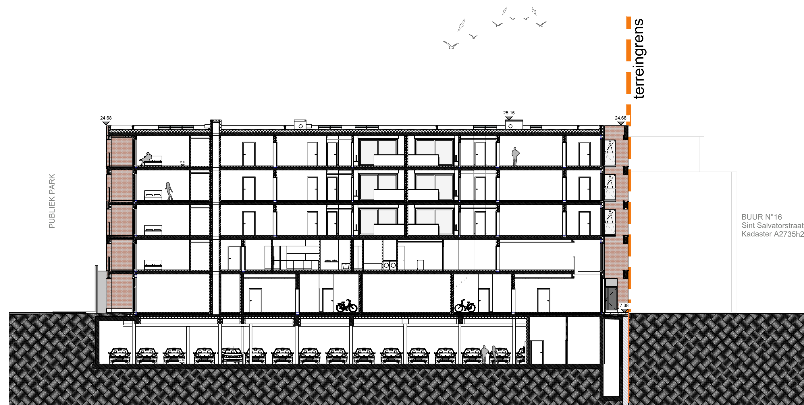
snede GG
