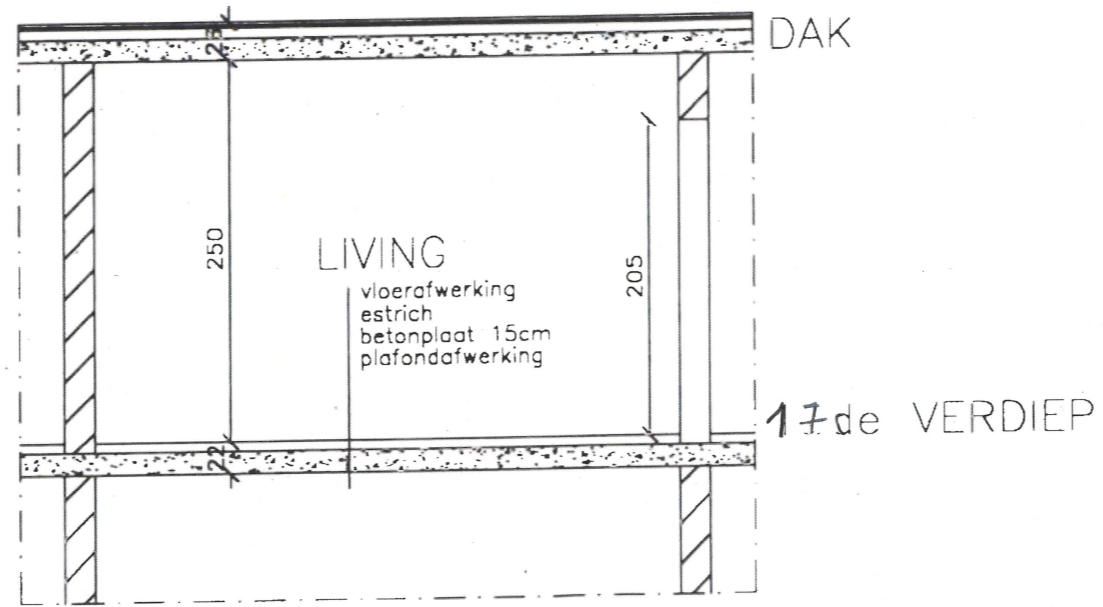
DOORSNEDE/AANZICHT 1-1
