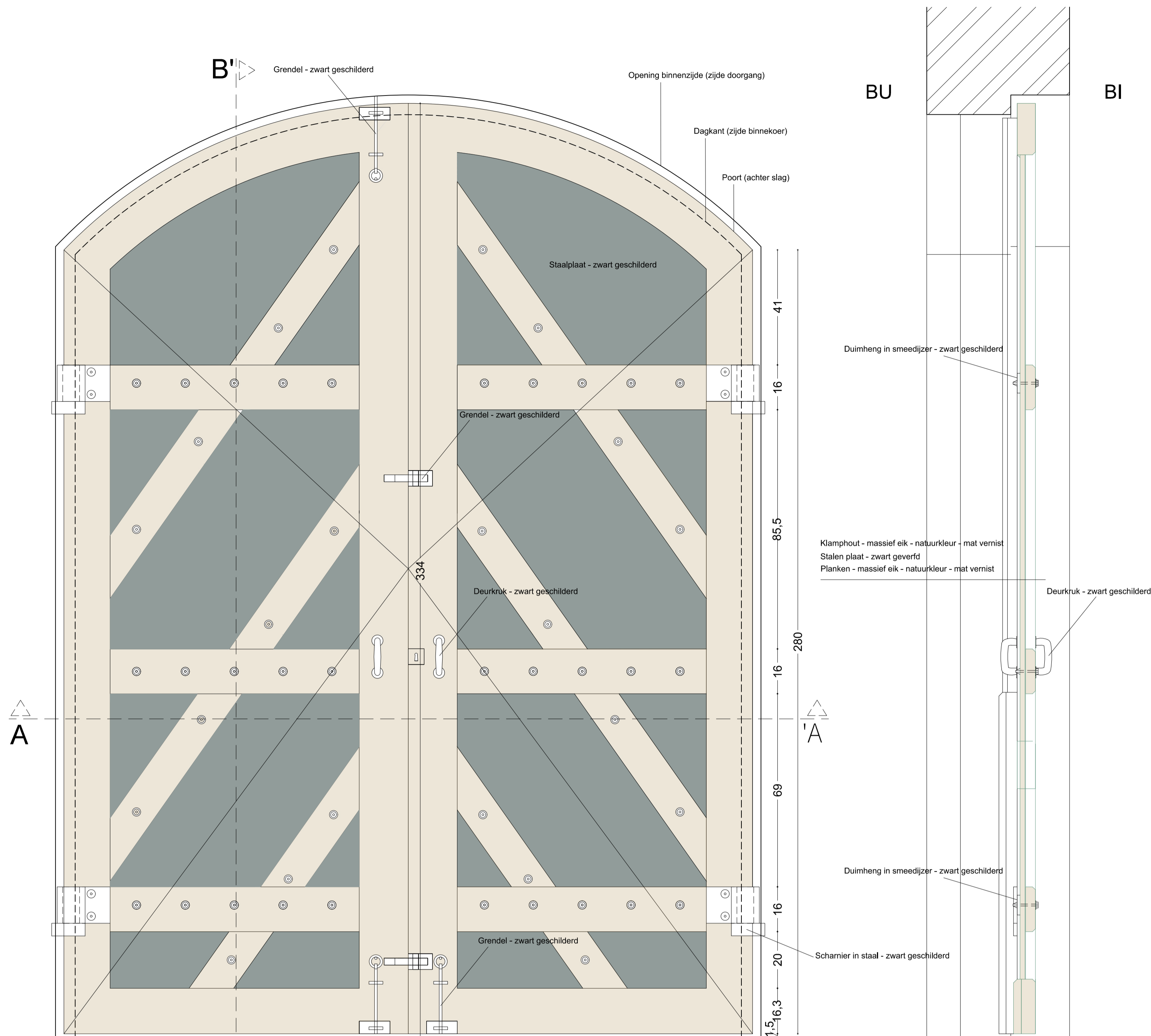
AANZICHT POORT (BINNENZIJDE - DOORGANG)
