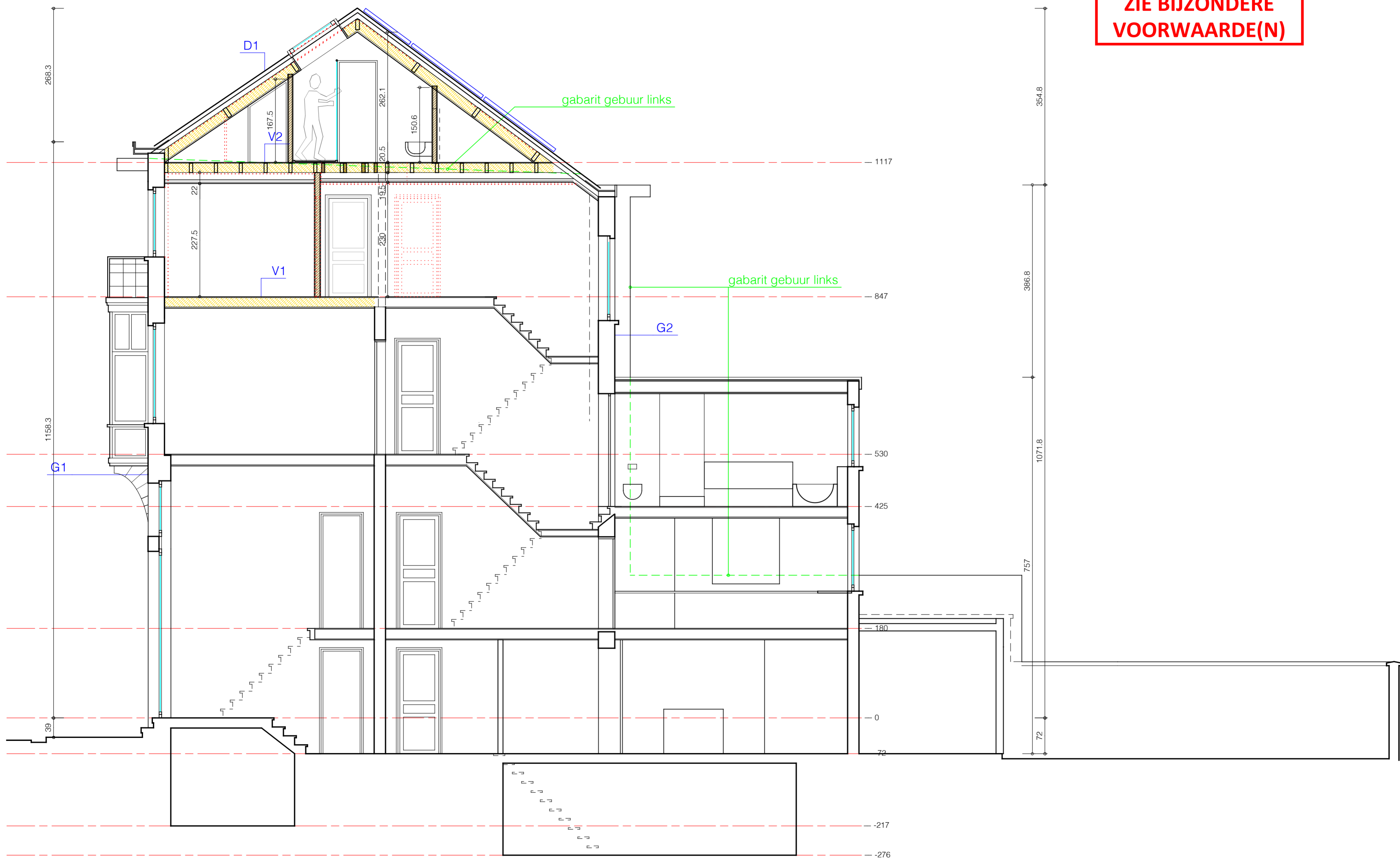
snede 2
