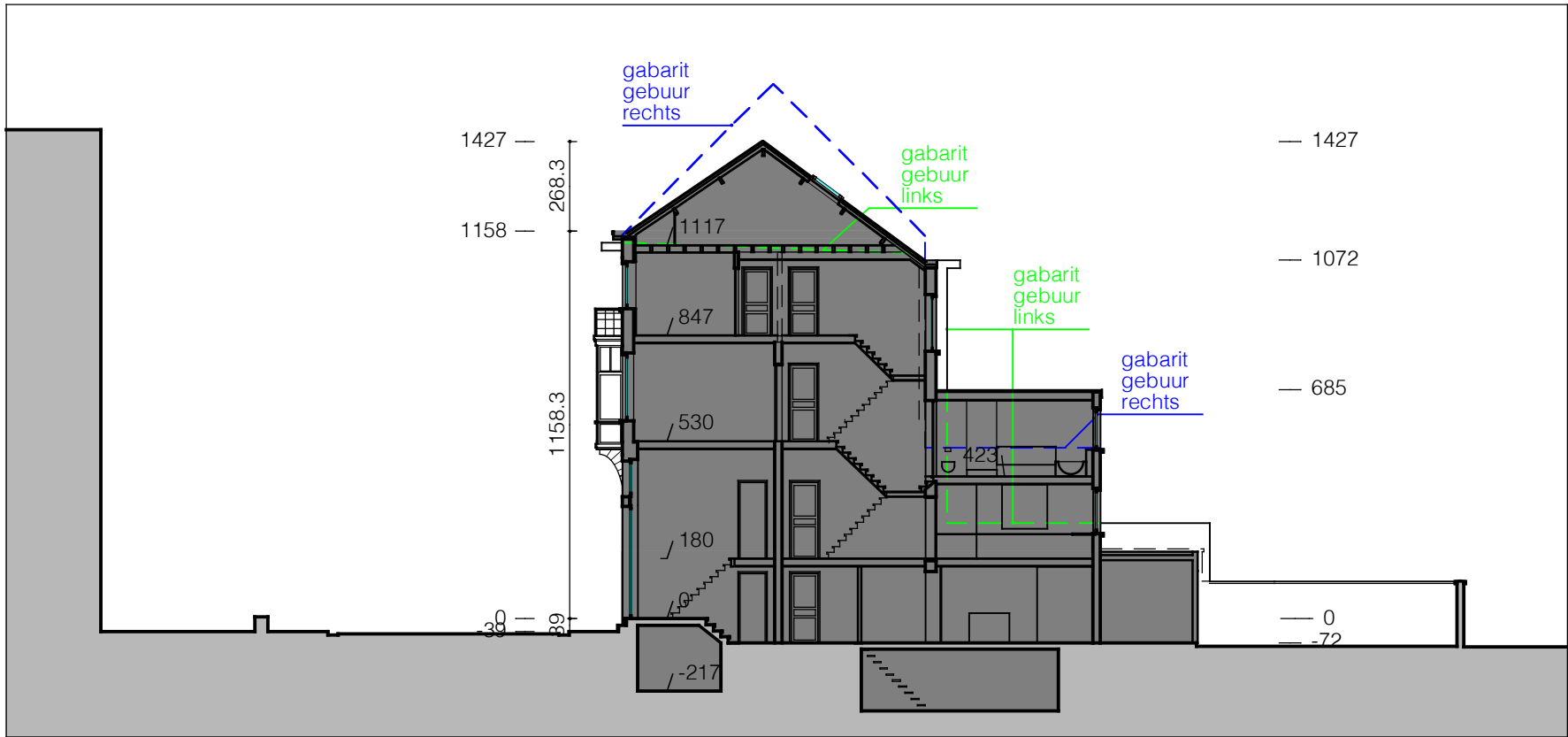
terreinprofiel - bestaande toestand
