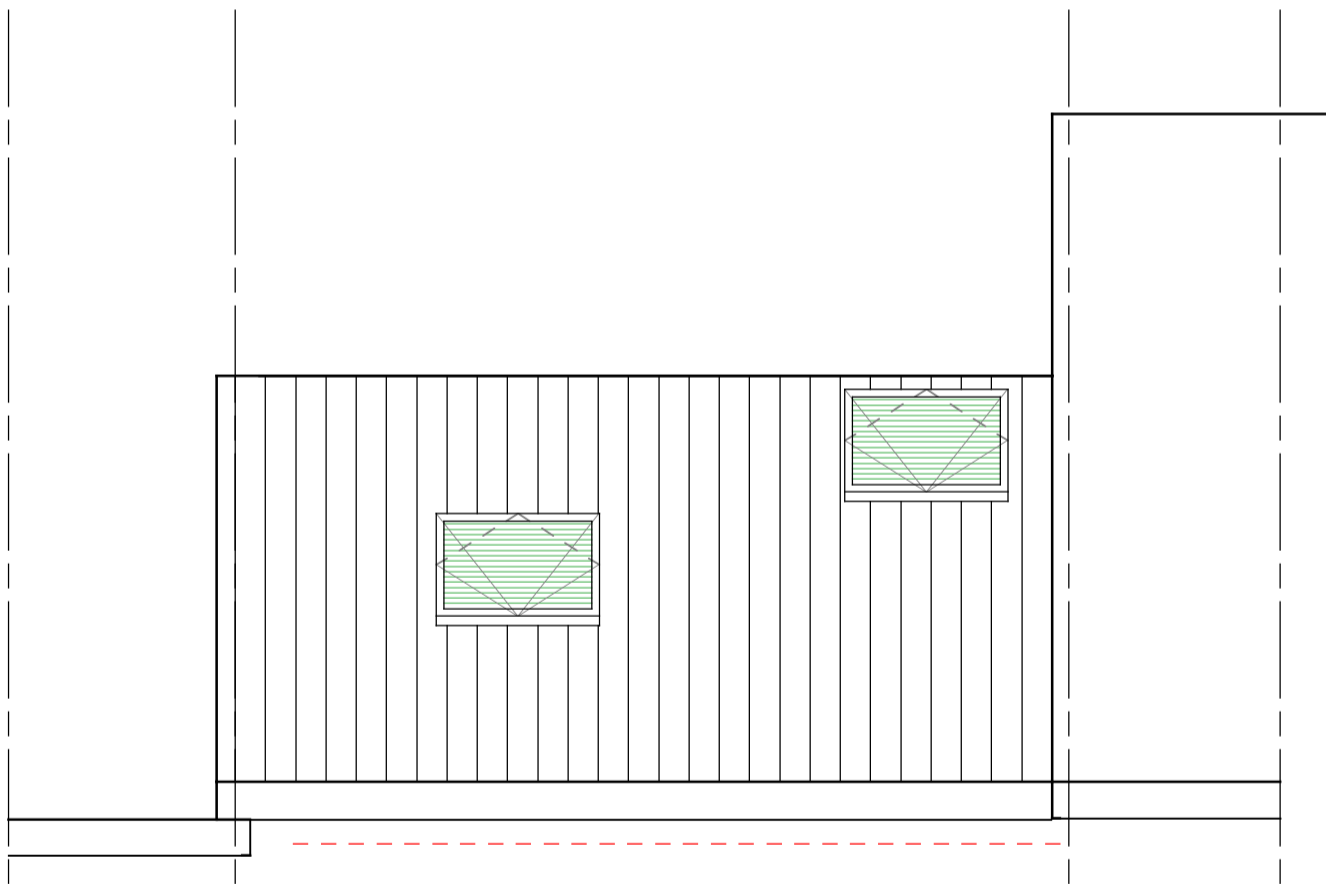
straatgevel fragment dak
