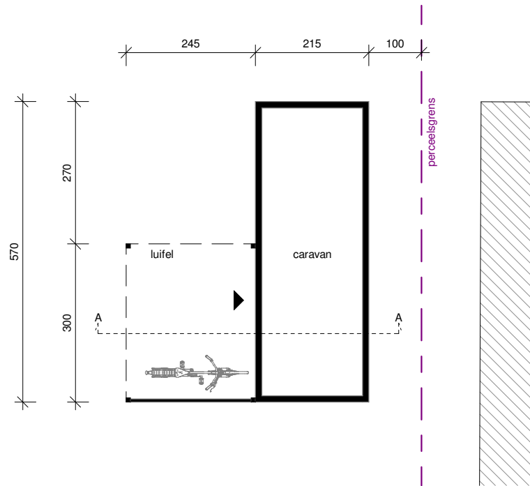
1 1 : 100 plan
