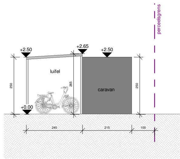
2 1 : 100 snede AA
