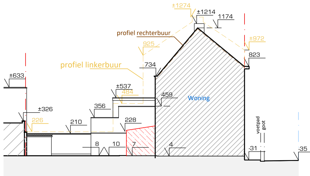
TERREINPROFIEL BESTAAND (sch. 1/200)
