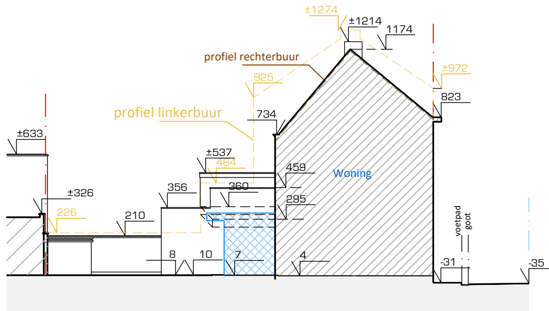
TERREINPROFIEL NIEUW (sch. 1/200)
