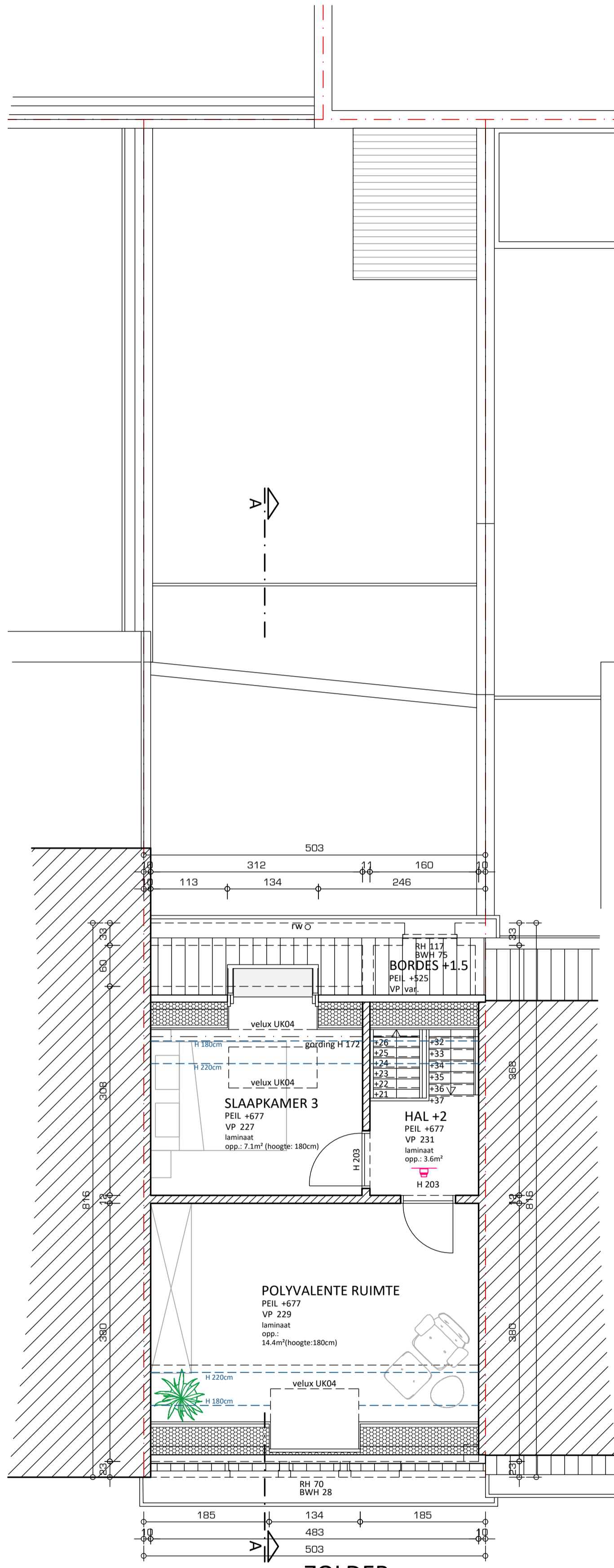
ZOLDER horizontale snede op H160cm (tov peil +677)
