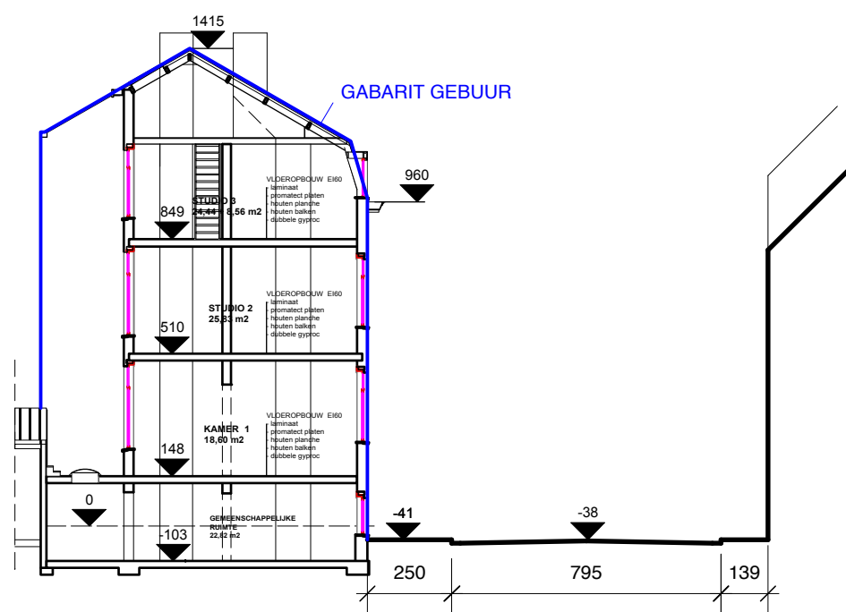
TERREINDOORSNEDE nieuwe toestand schaal 1/200
