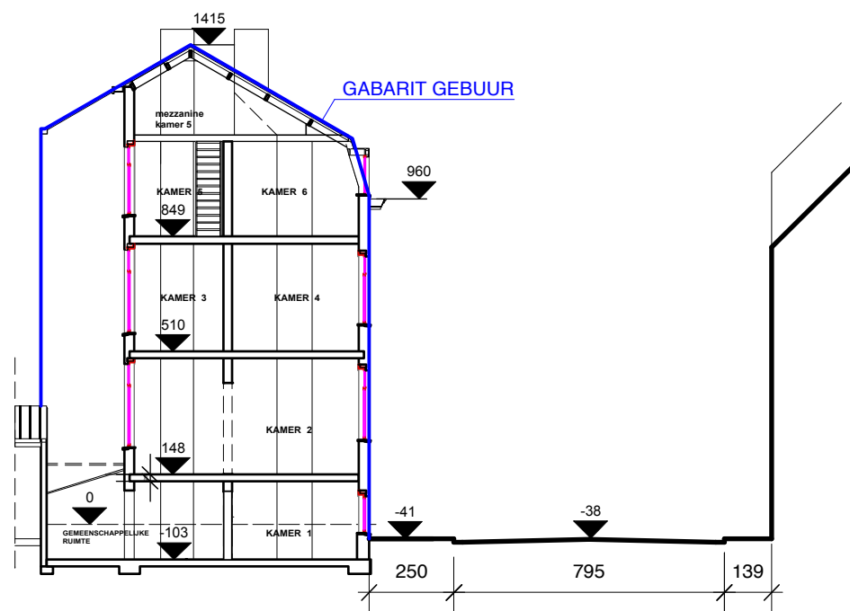
TERREINDOORSNEDE bestaende toestand schaal 1/200
