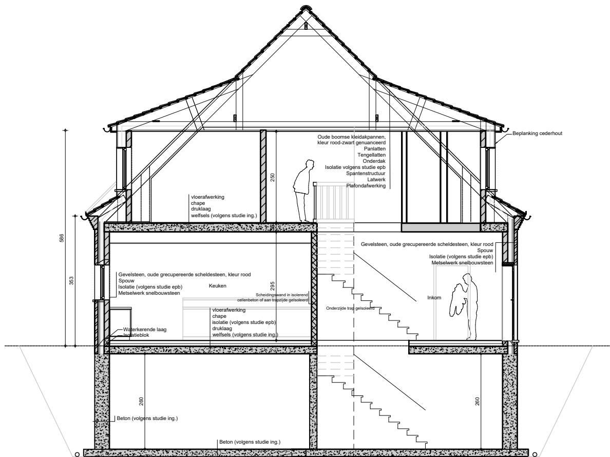
DOORSNEDE A-A NIEUWE TOESTAND
