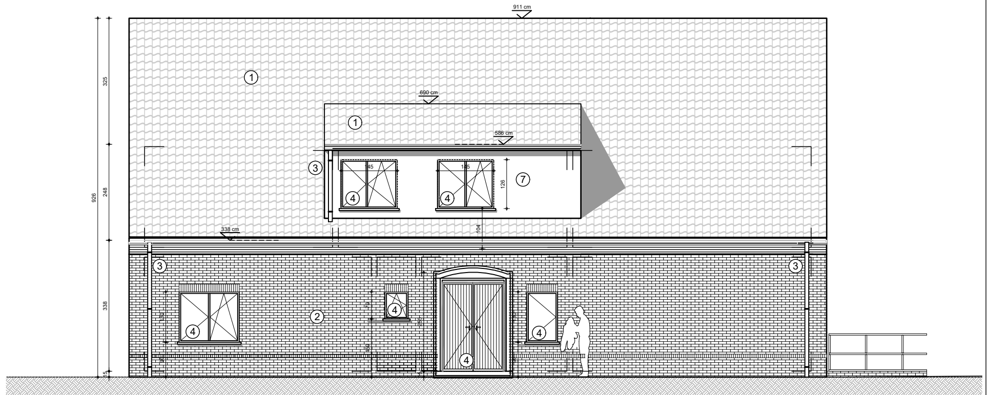
RECHTER ZIJGEVEL NIEUWE TOESTAND
