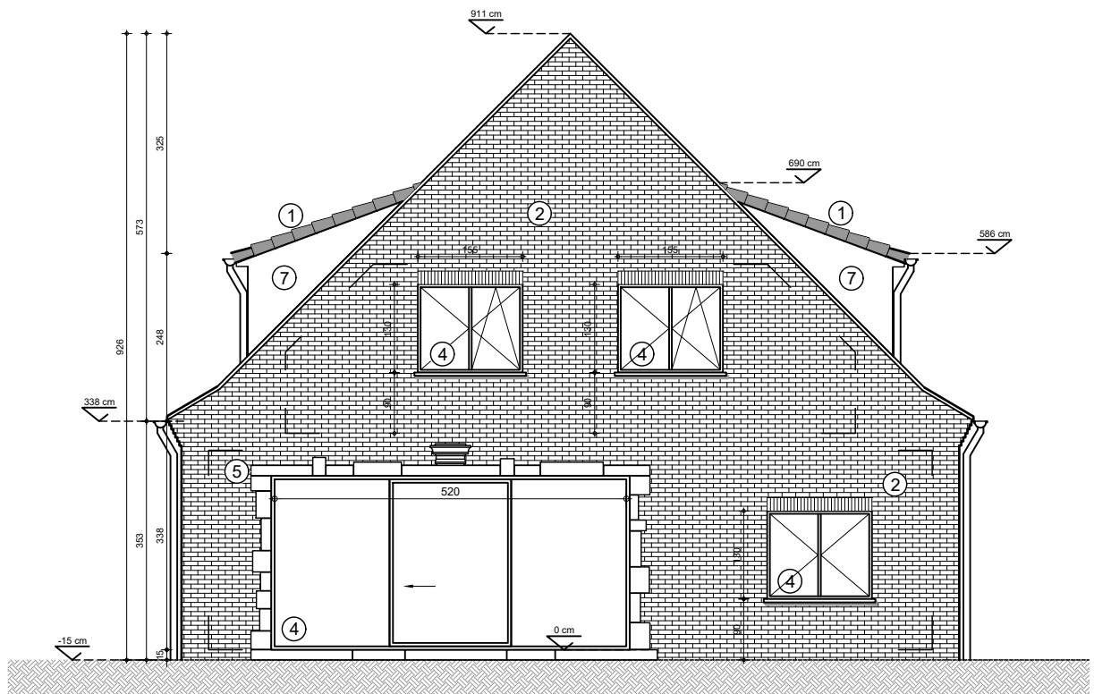
VOORGEVEL BESTAANDE TOESTAND
