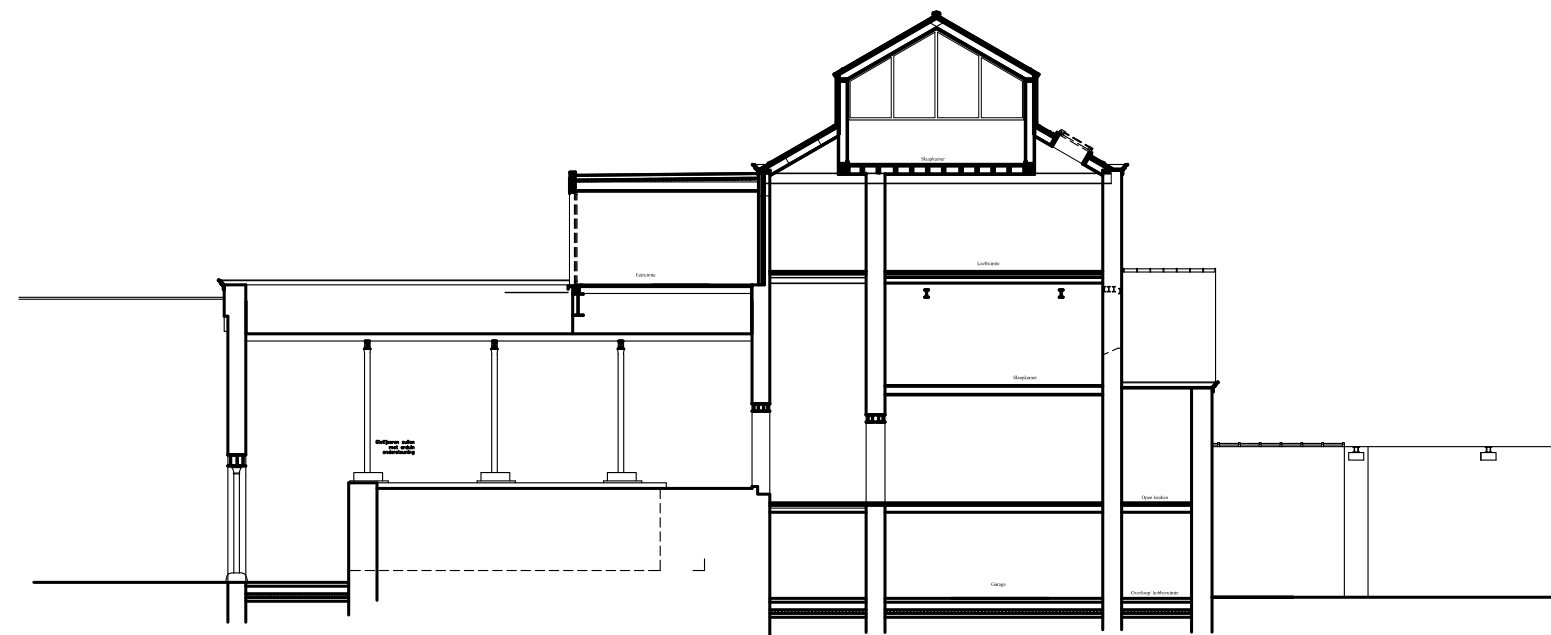
Terreinprofiel aa
