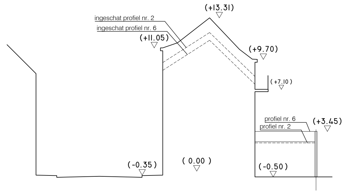
TERREINPROFIEL 1/200
