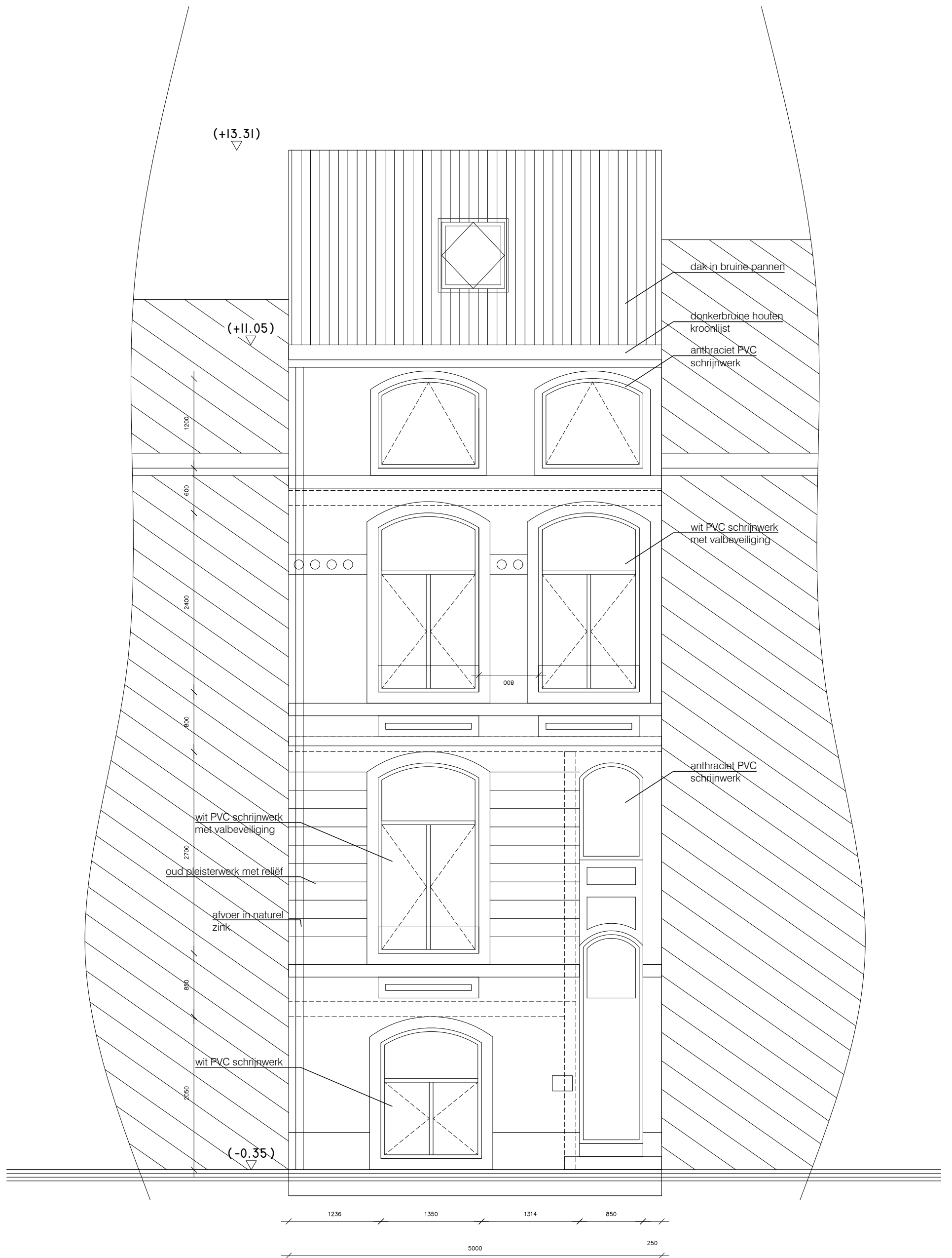
VOORGEVEL 1/50
