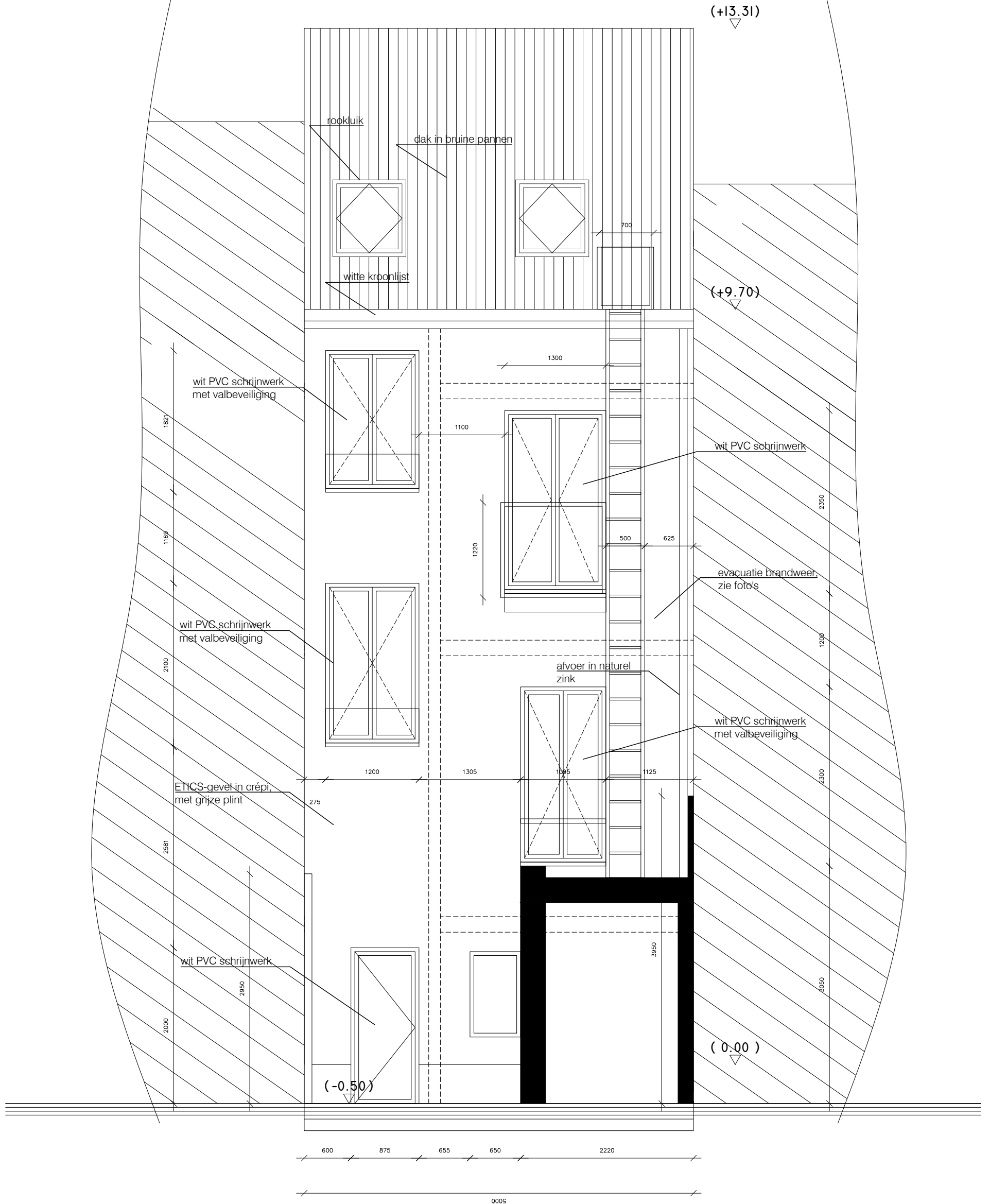
ACHTERGEVEL 1/50
