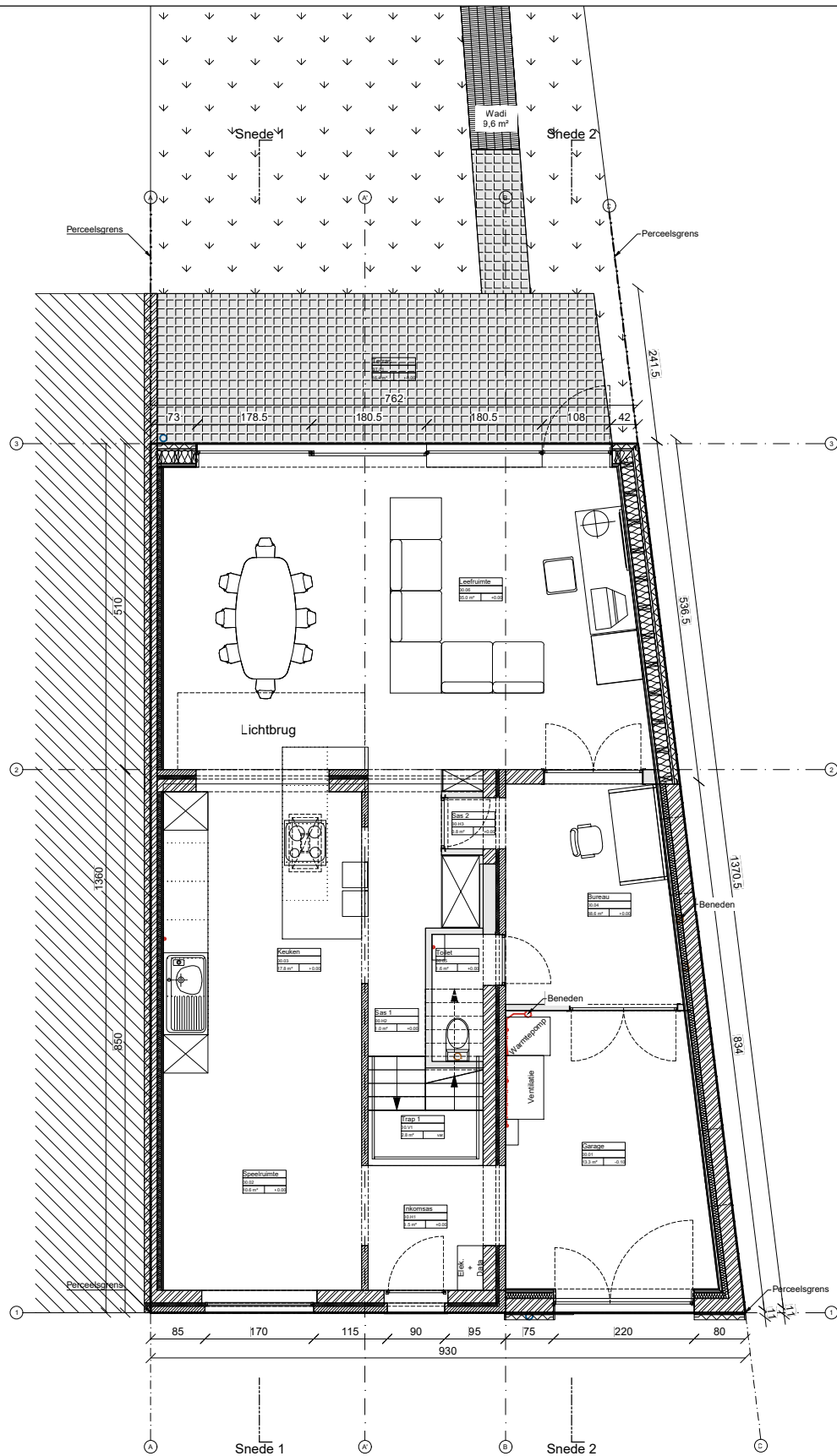
Grondplan +0
