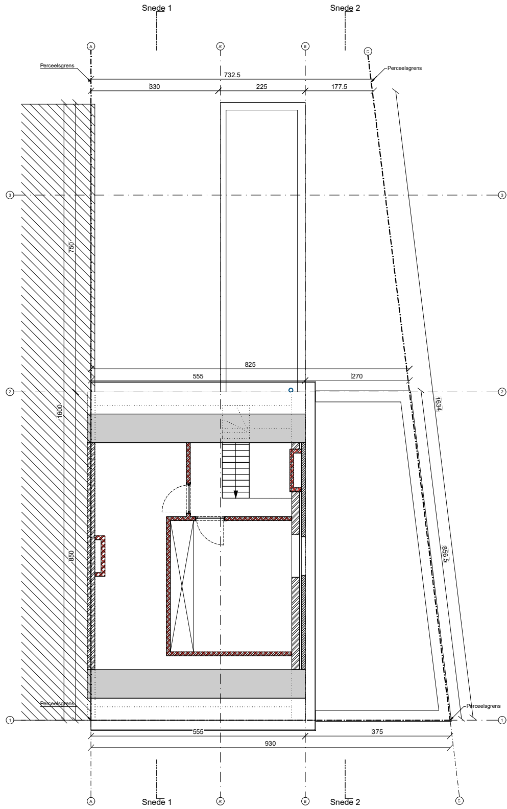
Grondplan +2
