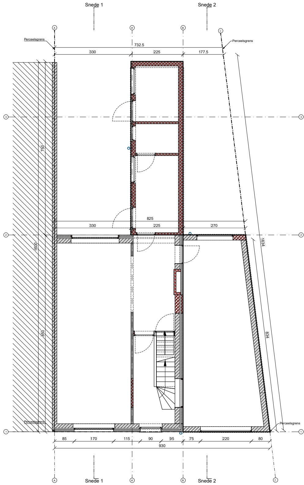
Grondplan +0
