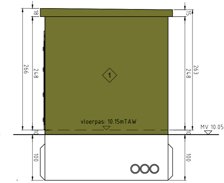
Rechteraanzicht
