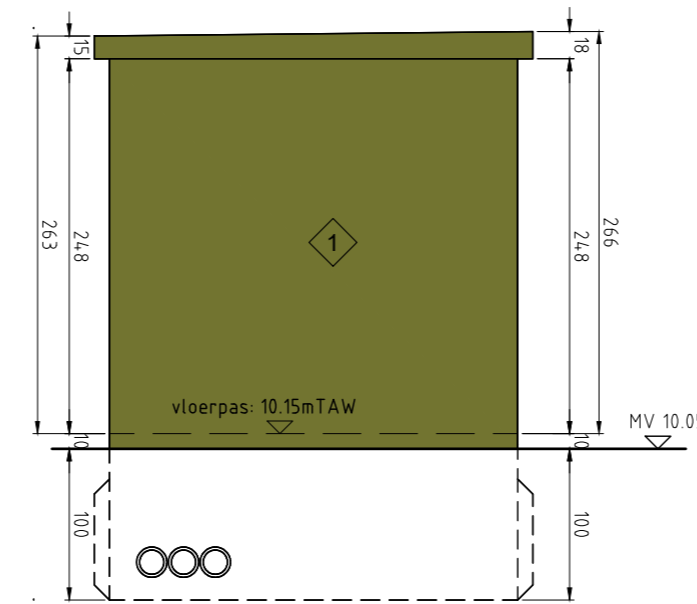
Linkeraanzicht
