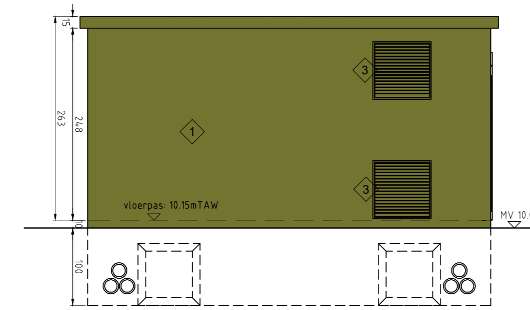
Achteraanzicht
