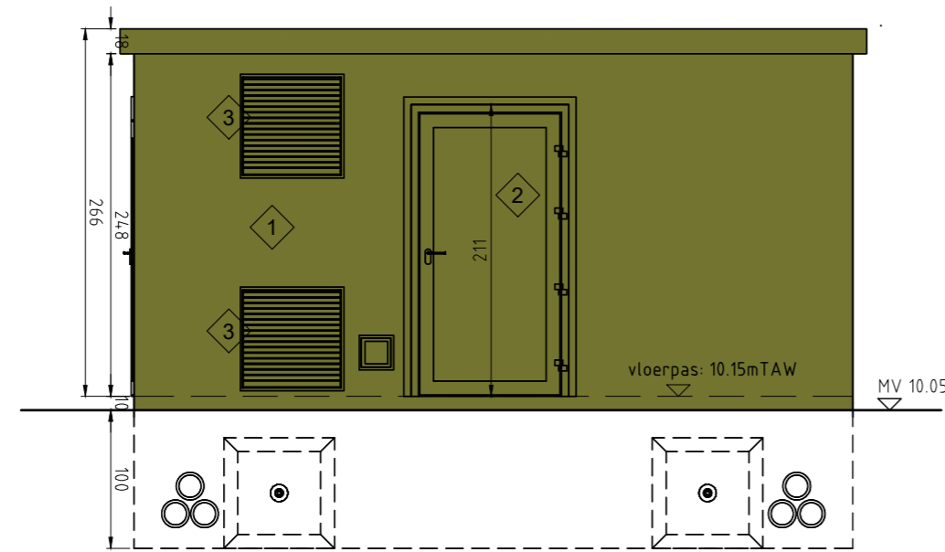
Vooraanzicht
