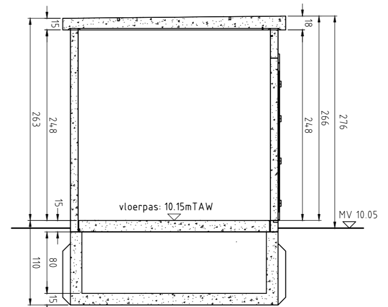
Snede S1
