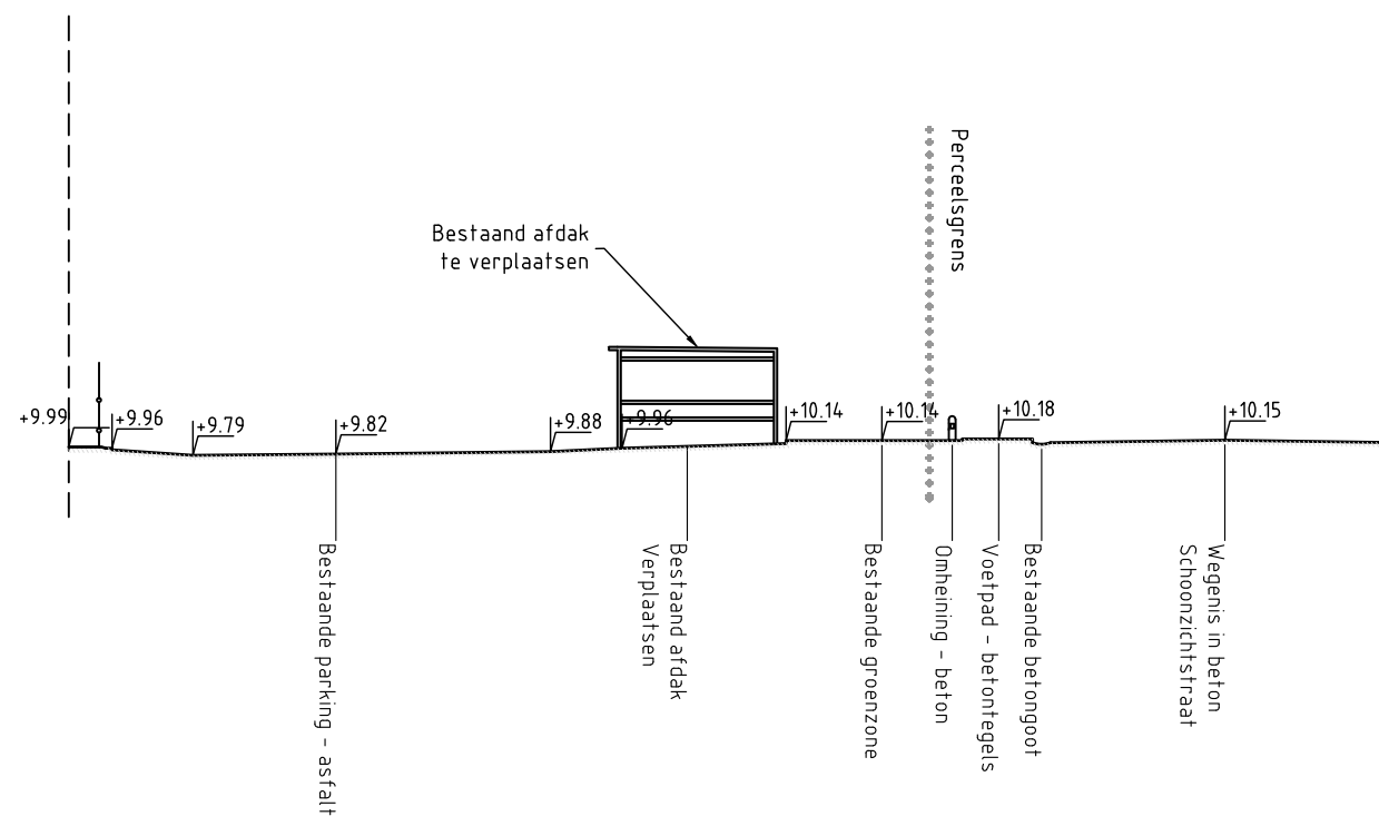
Terreinprofiel T1-Bestaande toestand
